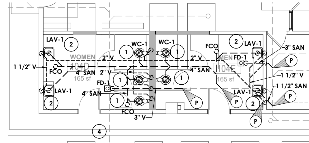
5 104D & 104E SAN & VENT NEW WORK P201 SCALE: 1/8" = 1'-0"
